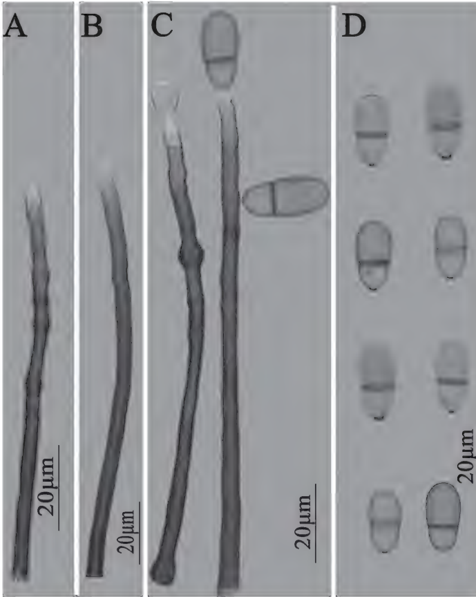
FIG. 4. Endophragmiella resiniae .
